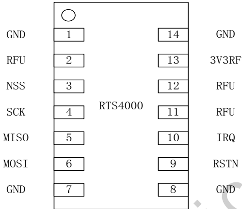
图 3-1 RTS4000 管脚图
