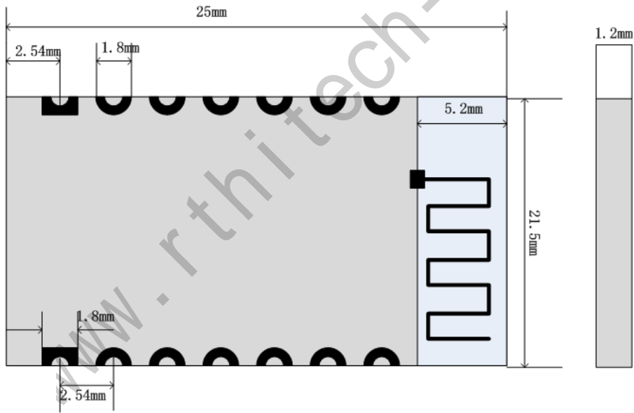
图 3-2 RTS4000 尺寸图
